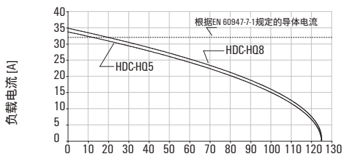
HDC-HQ5 和 HDC-HQ8 / H07V-K4.0
