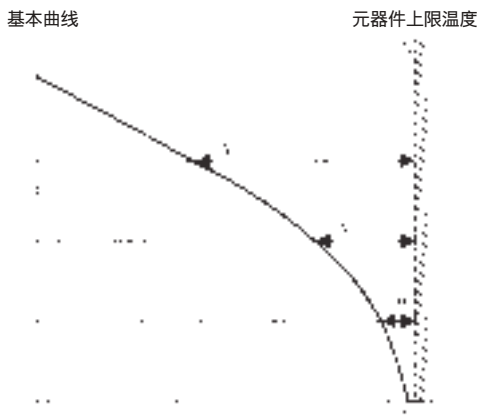
t_u = 元件上限温度 t_a = 环境温度 I_a = 电流
