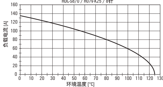
衰减曲线
