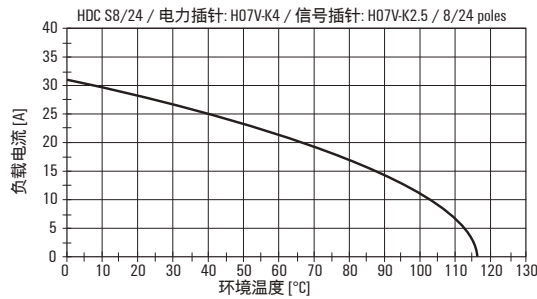
衰减曲线
