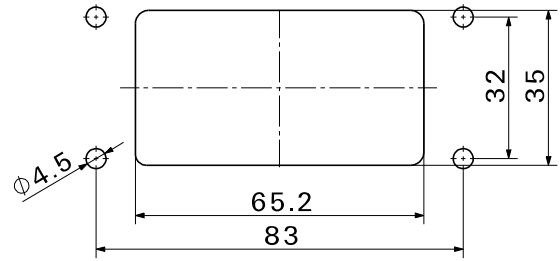
16 芯面板開孔尺寸圖
