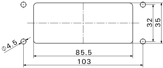
24 芯面板開孔尺寸圖
